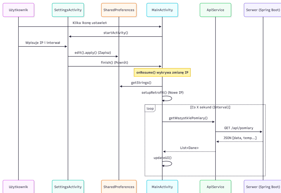
Rysunek 2. Diagram Sekwencji (Przepływ danych)
