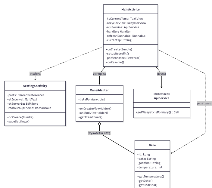
Rysunek 1. Diagram Klas (Struktura aplikacji)
